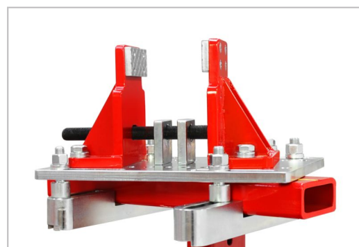
No.4 Pinces de seuil pour camionnettes et tout-terrains
